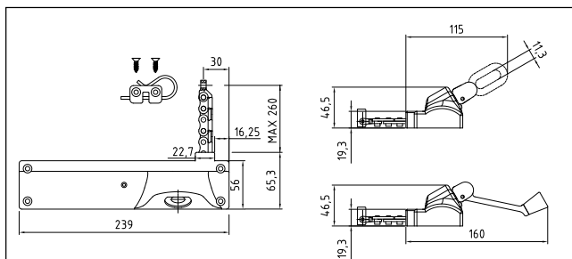
Dimensioni dell'attuatore
